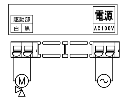
端子結線図
