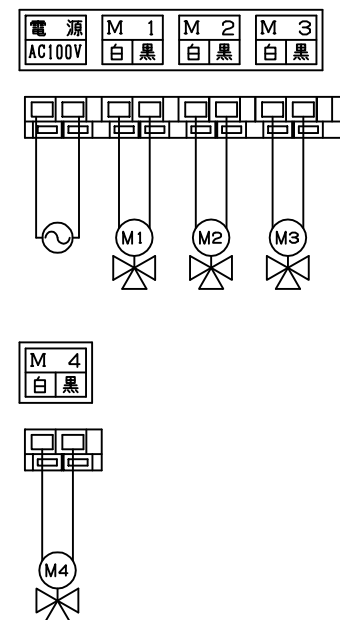
端子結線図
