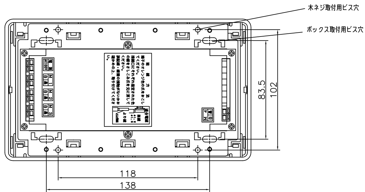
外形寸法図
