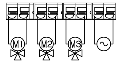
端子結線図
