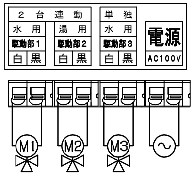
端子結線図
